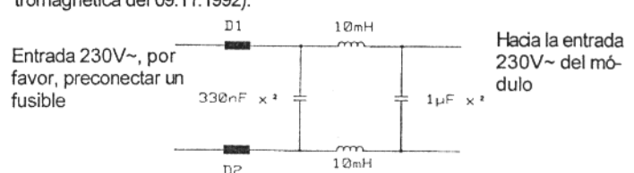
D1/D2 = Choque de banda ancha de VHF, 6-agujeros
