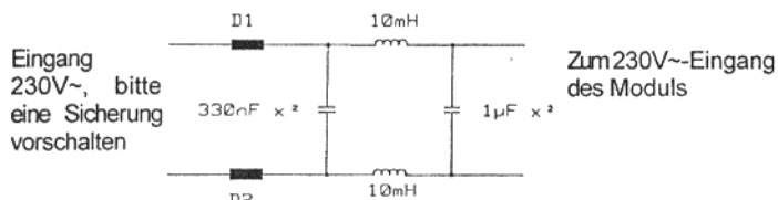
D1/D2 = 6-Loch-UKW-Breitbanddrossel
